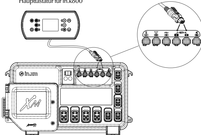
Haupttastatur für in.k800
